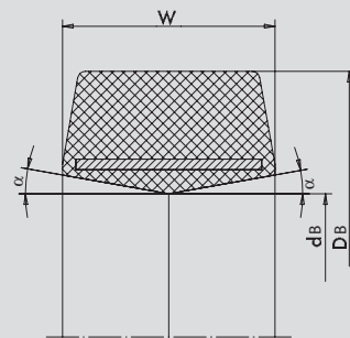
km = konischer Reifenfuß mittengeteilt (symmetrisch) km 15 = \alpha 15^\circ km 8 = \alpha 8^\circ
