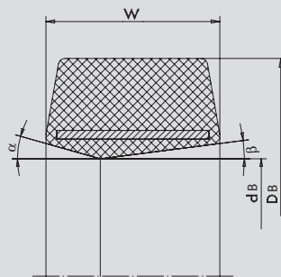
ks = konischer Reifenfuß seitengeteilt (asymmetrisch) ks 15/6 = \alpha 15^\circ, \beta 6^\circ ks 23/9 = \alpha 23^\circ, \beta 9^\circ
